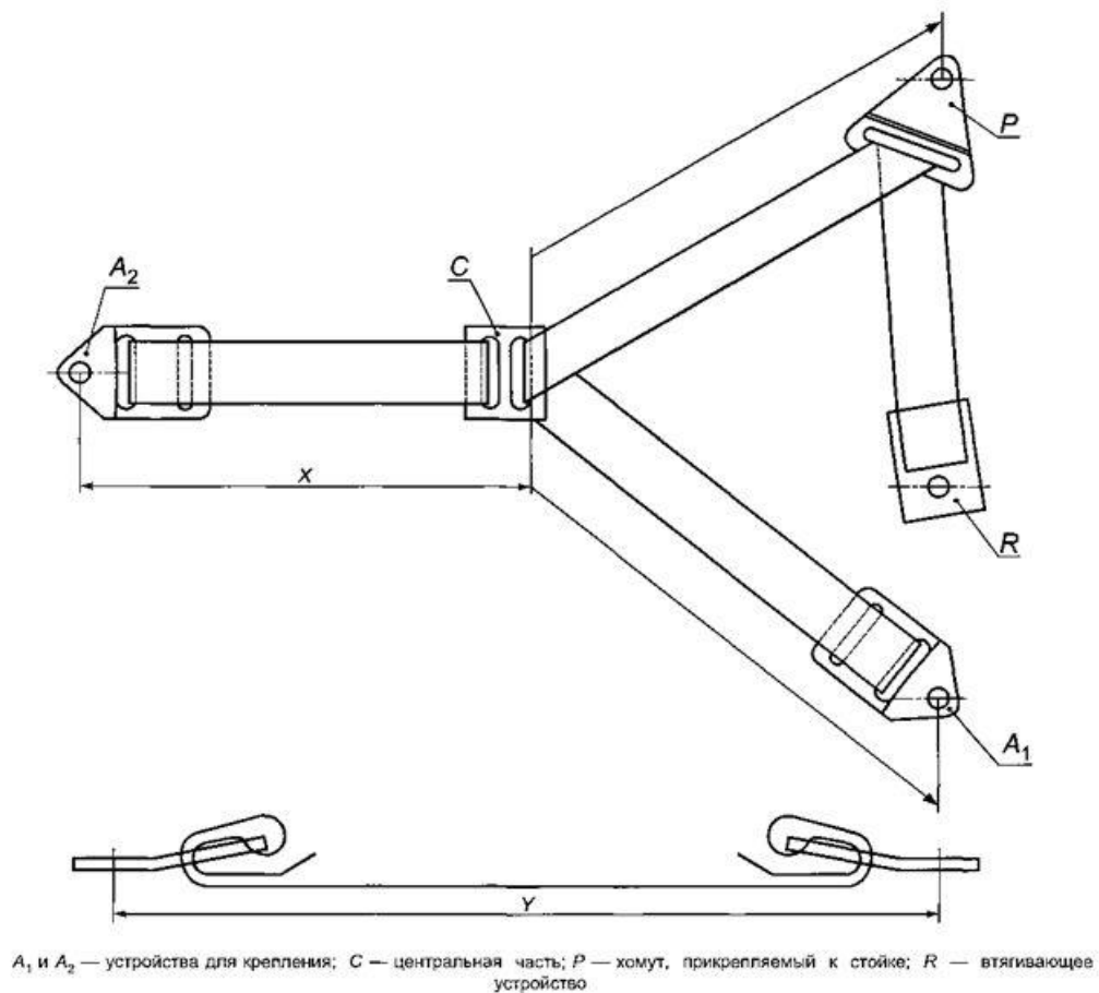
Рисунок П.1 — Конфигурация стандартного ремня безопасности
