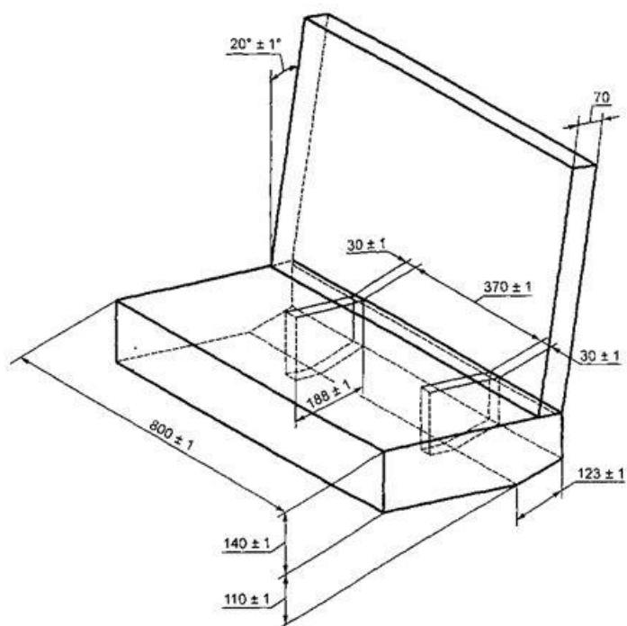
Рисунок Е 5 — Размеры сиденья (трехмерное изображение) Рис. Е.5. Размеры сиденья (трехмерное изображение)
